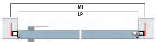
SEZIONE ORIZZONTALE
